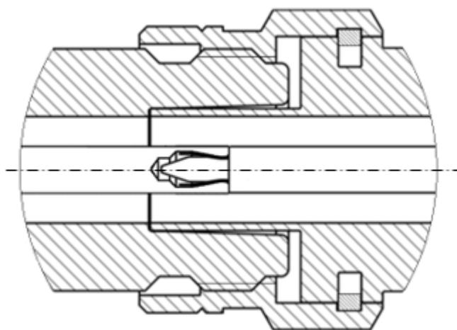
Рисунок 8 – Соединители тип N (розетка слева, вилка справа)
