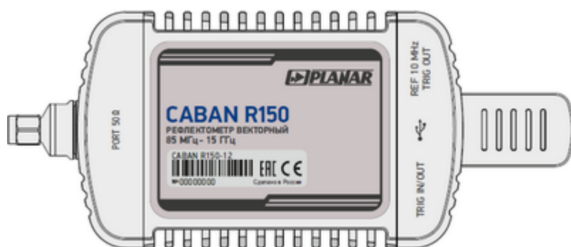
Рисунок 25 – Лицевая сторона
