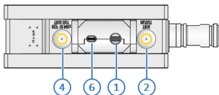
Рисунок 29 – Торцевая сторона
