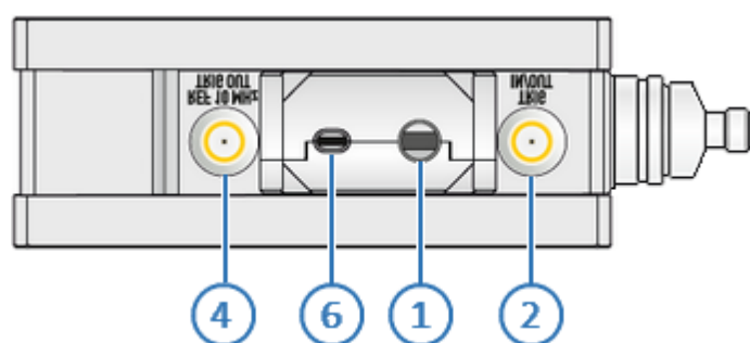
Рисунок 33 – Торцевая сторона
