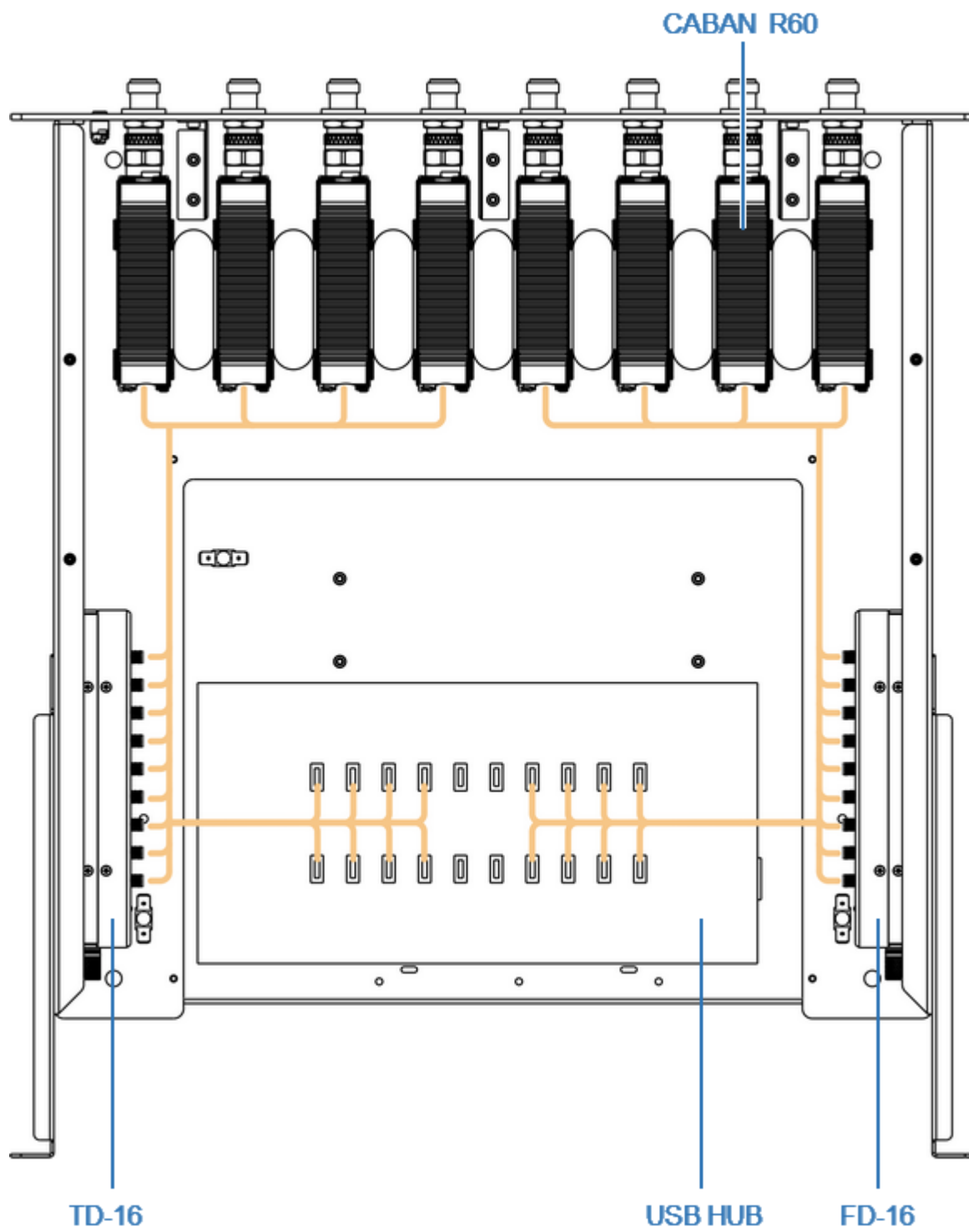
Рисунок 40 – Вид сверху
