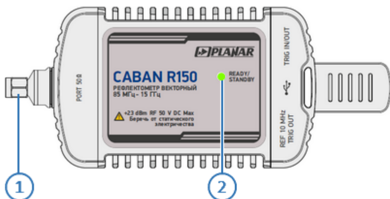
Рисунок 26 – Обратная сторона
