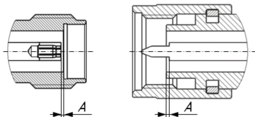
Рисунок 7 – Соединители тип 3,5 мм (розетка и вилка)
