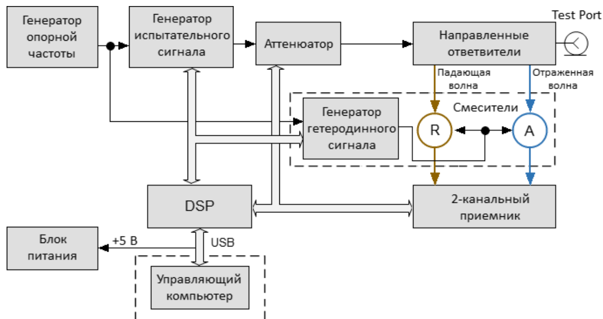
Рисунок 1 – Структурная схема рефлектометра векторного
