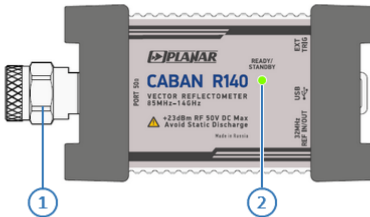
Рисунок 37 – Обратная сторона
