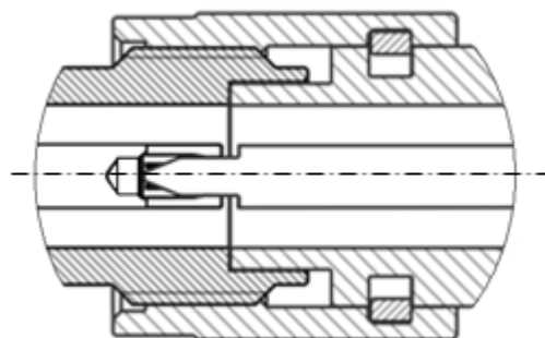
Рисунок 9 – Соединители тип 3,5 мм (розетка слева, вилка справа)
