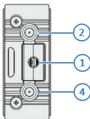
Рисунок 27 – Торцевая сторона
